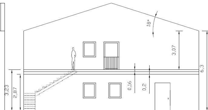
ANSICHT SÜD
