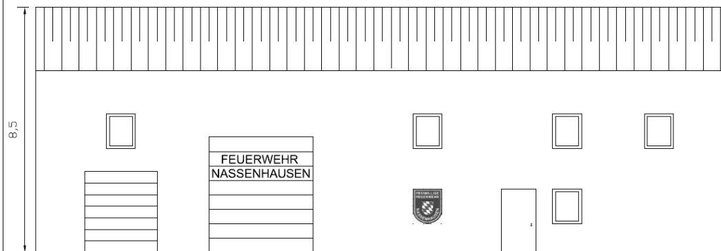
ANSICHT WEST
